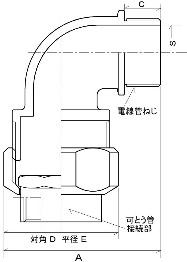
AG (厚鋼電線管用)
