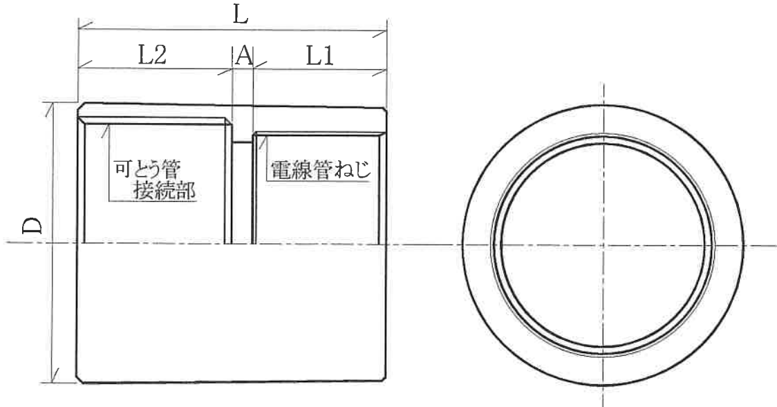
KC (薄鋼電線管用)
